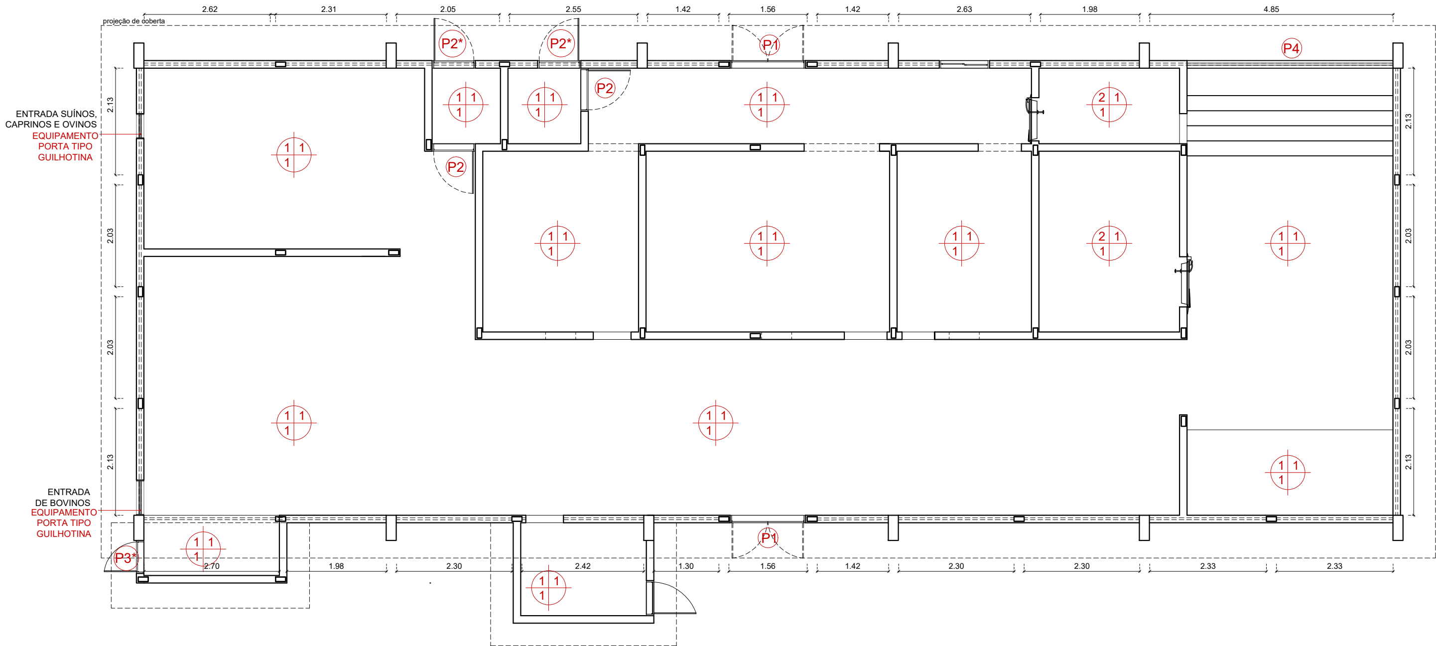
Planta Baixa Acabamento e esquadrias escala 1/75
