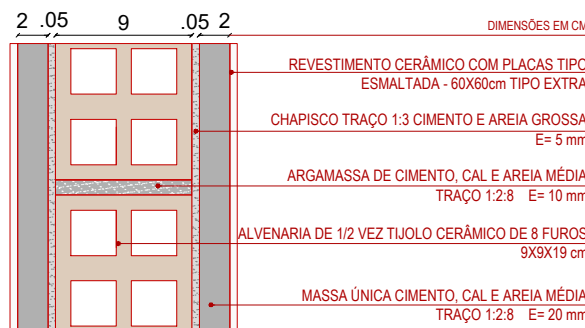
Detalhe - Alvenaria com revestimento escala 1/5
