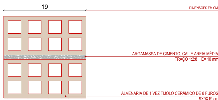
Detalhe - Fundação alvenarias galpão escala 1/5
