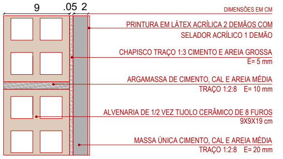
Detalhe - Alvenaria externa e das câmaras escala 1/5
